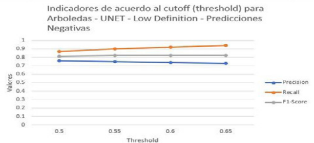
Fig. 5. Indicadores de acuerdo al threshold para Arboledas - U-Net - Low Definition - Predicciones Negativas
