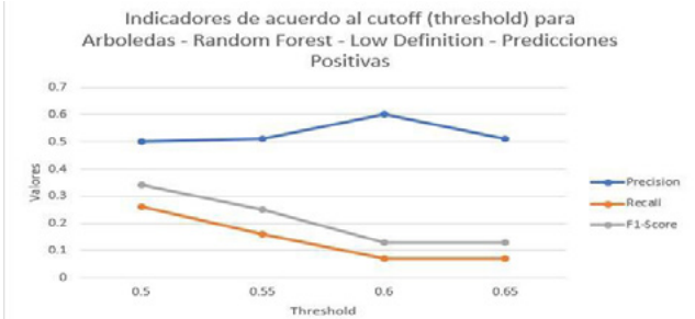
Fig. 4. Indicadores de acuerdo al threshold para Arboledas - Random Forest - Low Definition - Predicciones Positivas
